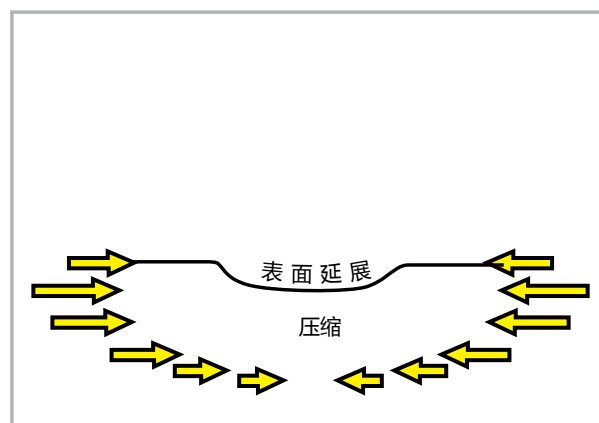
ABP形成的压应力
